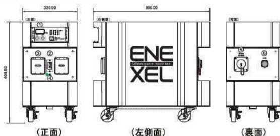
外観寸法 (単位:mm)
